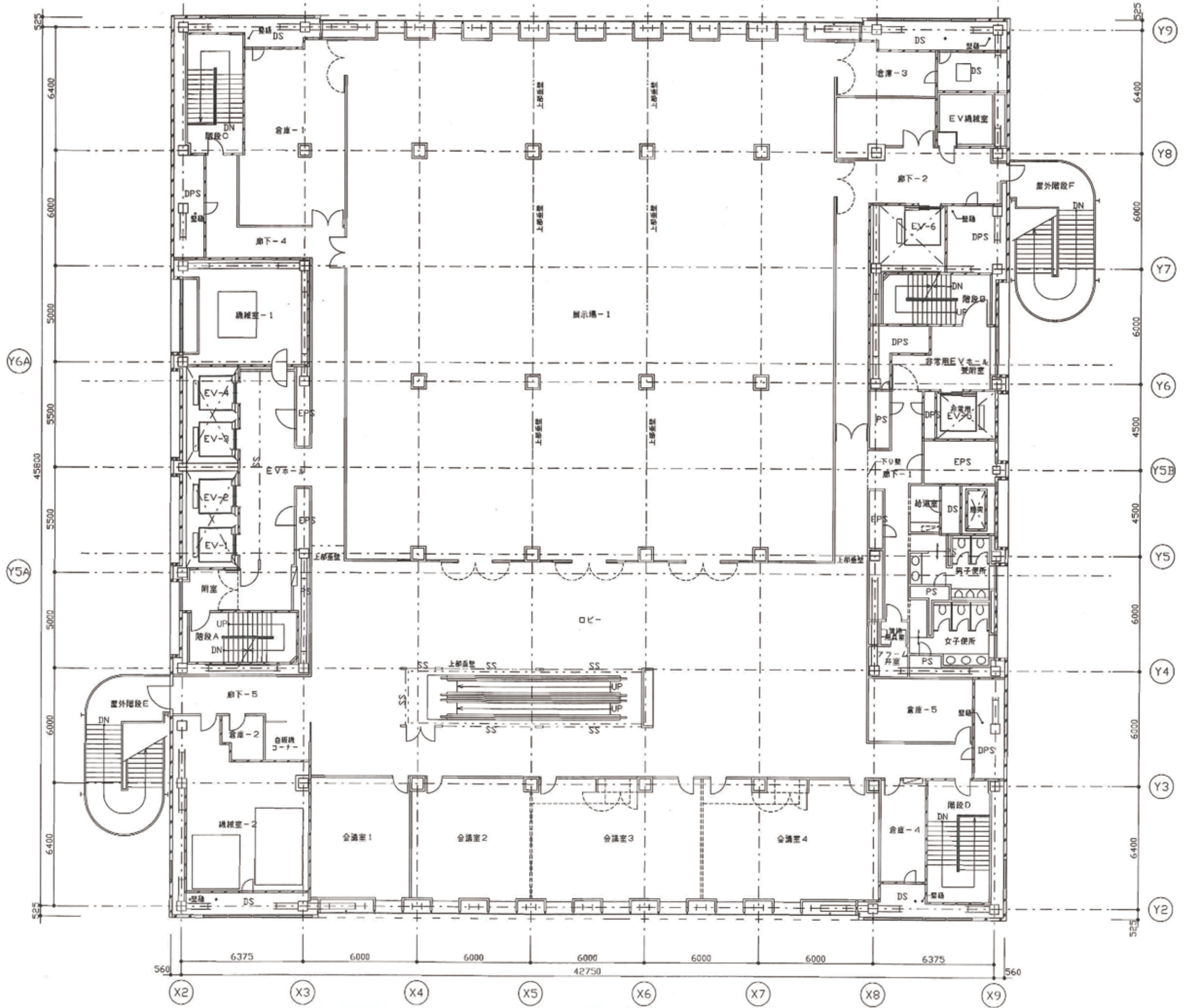
3階平面図 1/100
